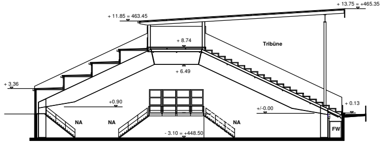
Querschnitt Ost
