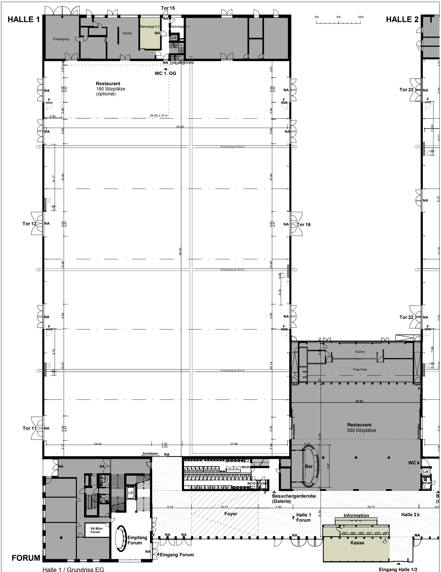
Halle 1 / Grundriss EG
