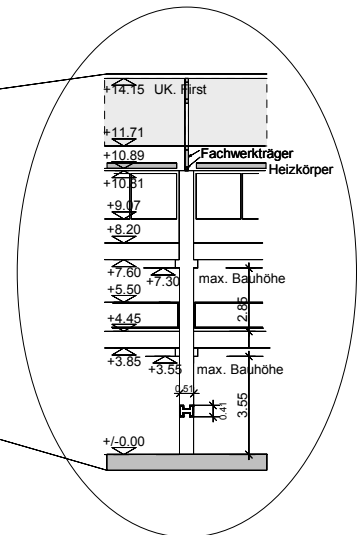
Detailansicht Schemaschnitt A-A (vergrössert)
